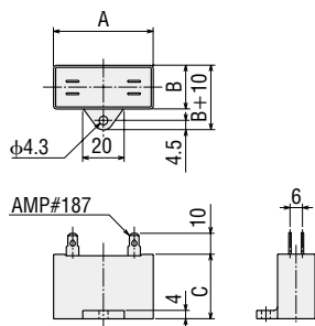
◇電容器外形尺寸表
