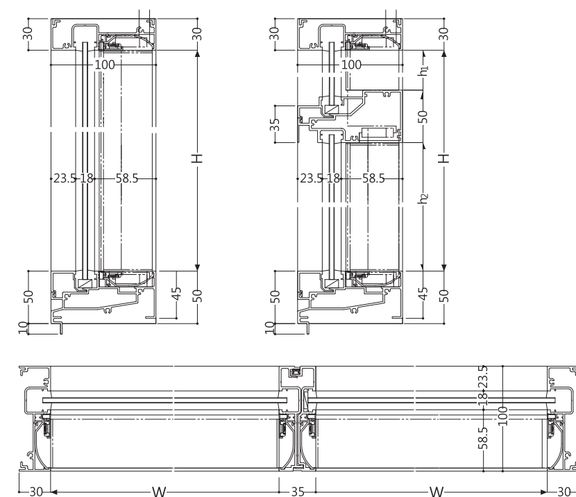
ALBEAM發光型門廳窗系統(FIX窗為例)
