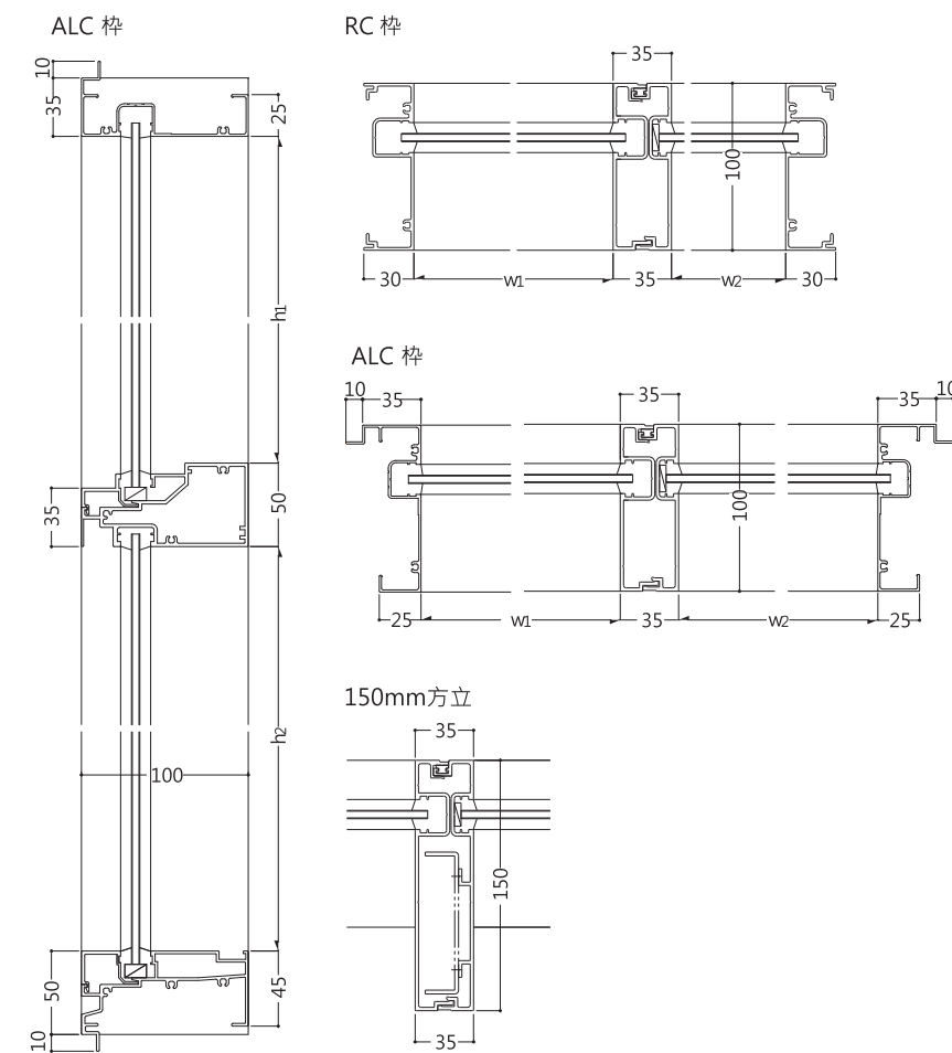
ALBEAM發光型門廳窗系統(FIX窗為例)
